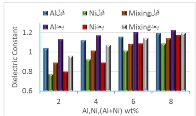
الشكل (4) مقارنة قيم ثابت العزل الكهربائي مع النسبة المئوية الوزنية لعينات الألمنيوم والنيكل والمزيج قبل وبعد التشعيع بالأشعة فوق البنفسجية
