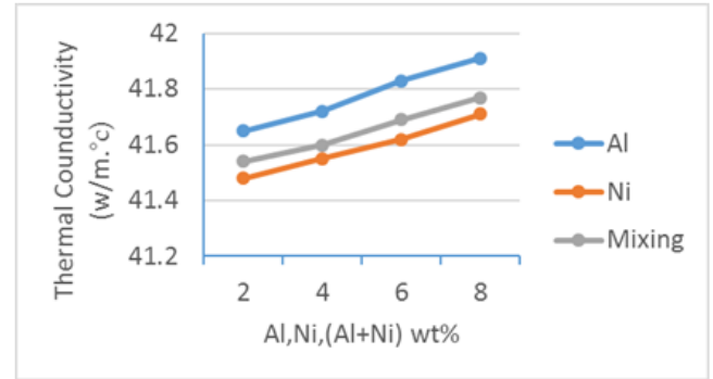
الشكل (6) مقارنة قيم التوصيلية الحرارية مع النسبة المئوية الوزنية لعينات الالمنيوم والنيكل والمزيج (المنيوم+نيكل) بعد التشعيع بالأشعة فوق البنفسجية
