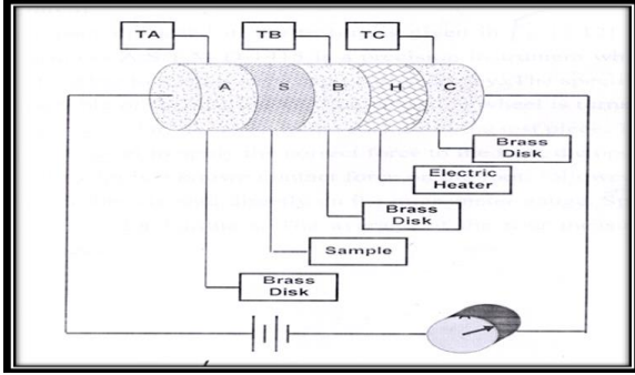
الشكل (1) مخطط جهاز التوصيلية الحرارية (قرص لي) [12]
