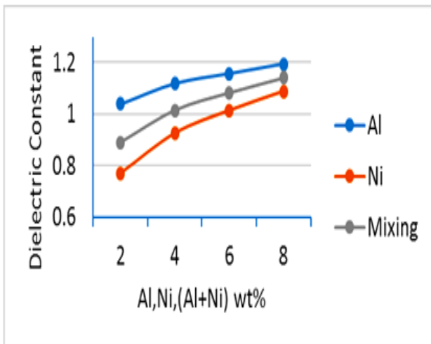
الشكل (2) مقارنة قيم ثابت العزل الكهربائي مع النسبة المئوية الوزنية لعينات الالمنيوم والنيكل والمزيج في الظروف الطبيعية
