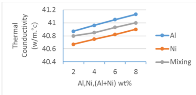
الشكل (5) مقارنة قيم التوصيلية الحرارية مع النسبة المئوية الوزنية لعينات الألمنيوم والنيكل والمزيج (المزيج+نيكل) في الظروف الطبيعية
