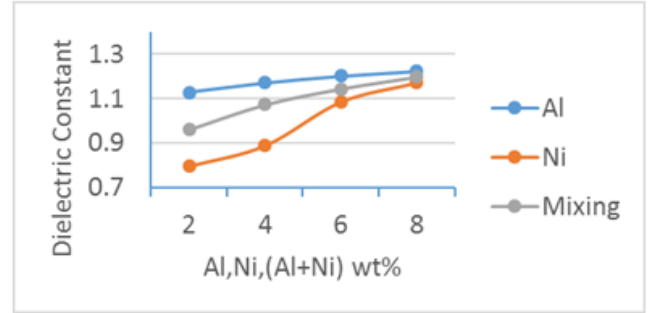
الشكل (3) مقارنة قيم ثابت العزل الكهربائي مع النسبة المئوية الوزنية لعينات الألمنيوم والنيكل والمزيج بعد التشعيع بالأشعة فوق البنفسجية
